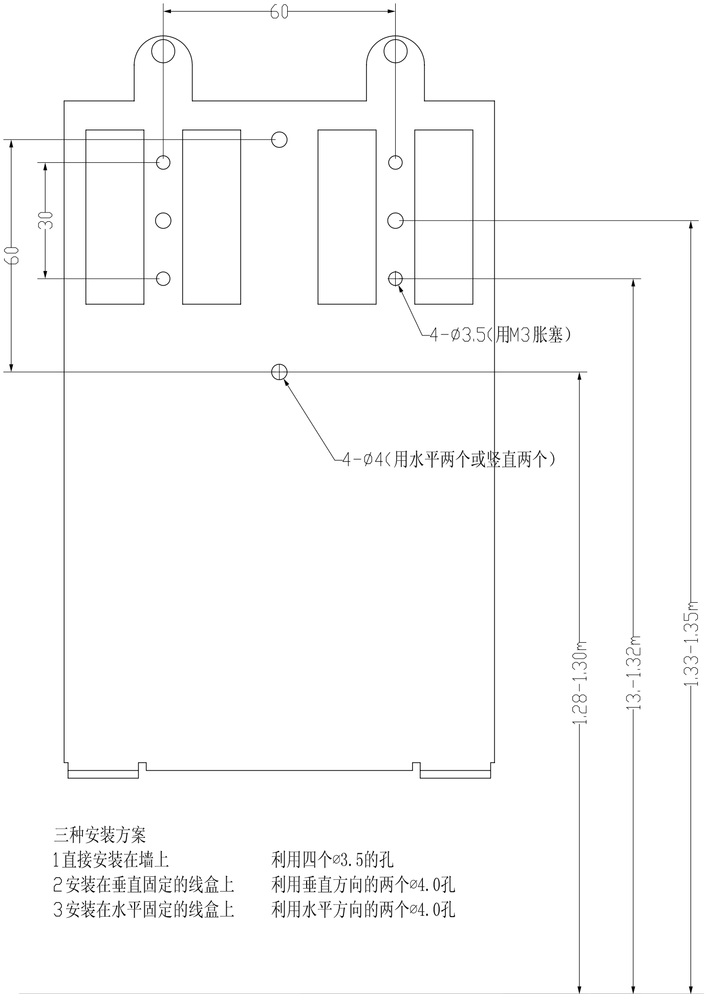
人脸识别机安装示意图
