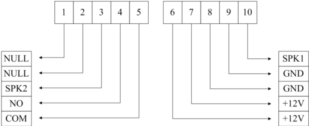
E390A端子图 GND：接地线；+12V：接12V输入电源；可用来替代标配电源适配器； NO、COM：继电器输出； SPK1、SPK2：接音频输出设备。
