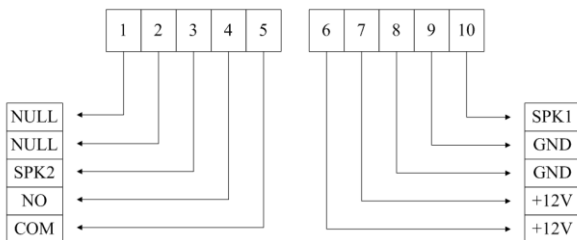
E390A端子图
