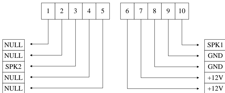
E352端子图
