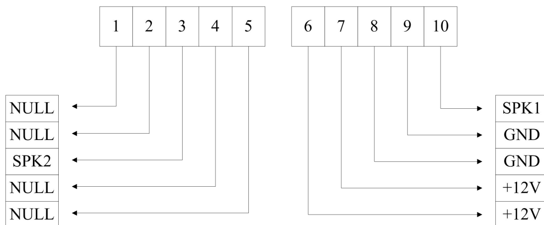
C330端子图
