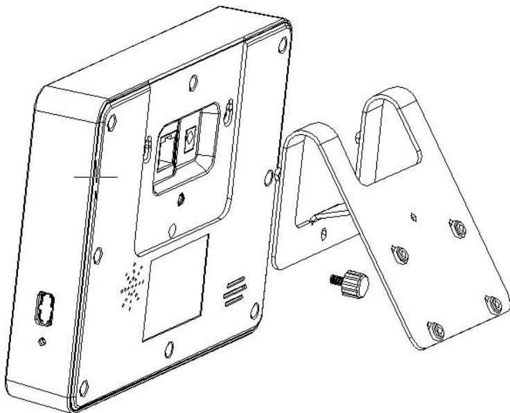
设备安装示意图
